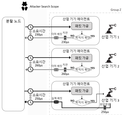
(그림 5) 지연을 통한 공격자 기만 방법
